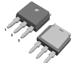
TO-251-3L 4N65D
